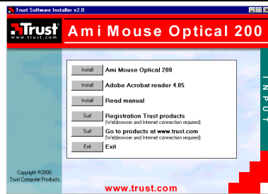
Abbildung 2: Software Installer
