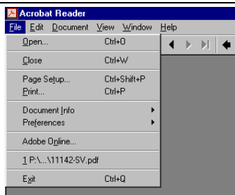
Abbildung 3: Datei öffnen
