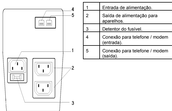
Figura 1: Conexões UPS
