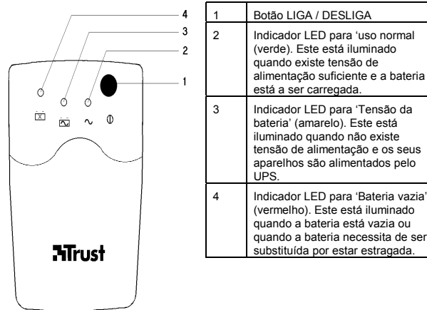
Figura 2: Funções UPS
