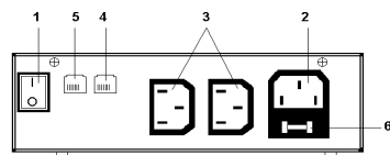
Figura 1: conexiones del UPS
