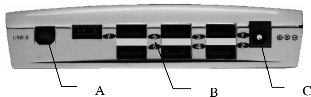
Figura 2: Face traseira do aparelho
