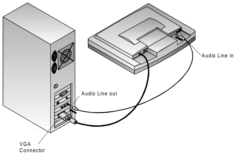
Figura 1: Collegamento del cavo VGA e del cavo audio
